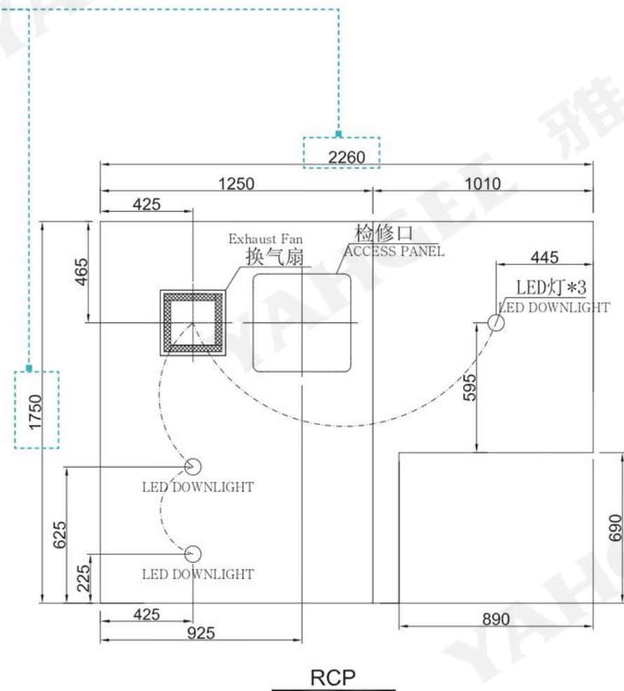
顶部布置图
