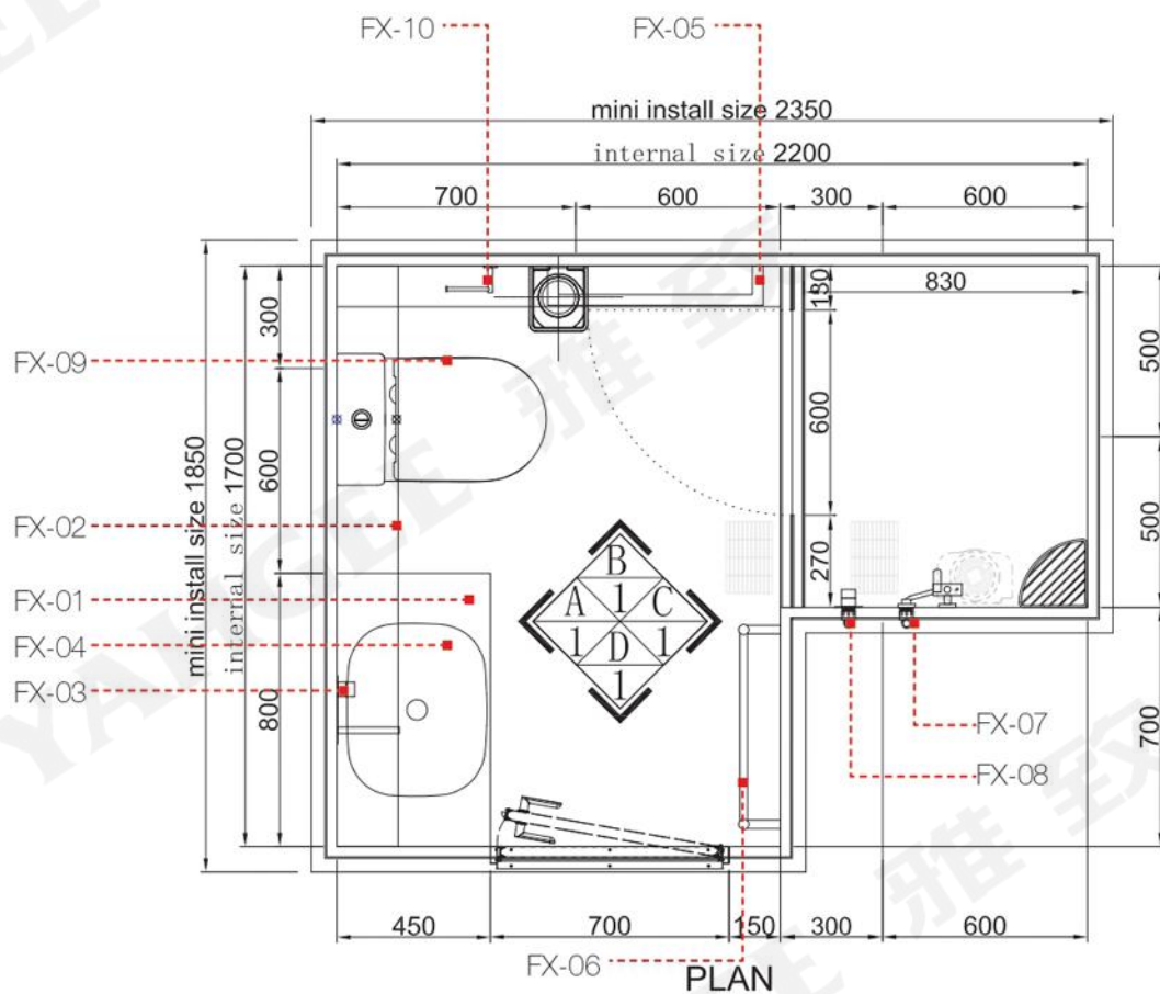
浴室平面布置图
